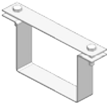
Kẹp nắp thang máng cáp Cover clamp
